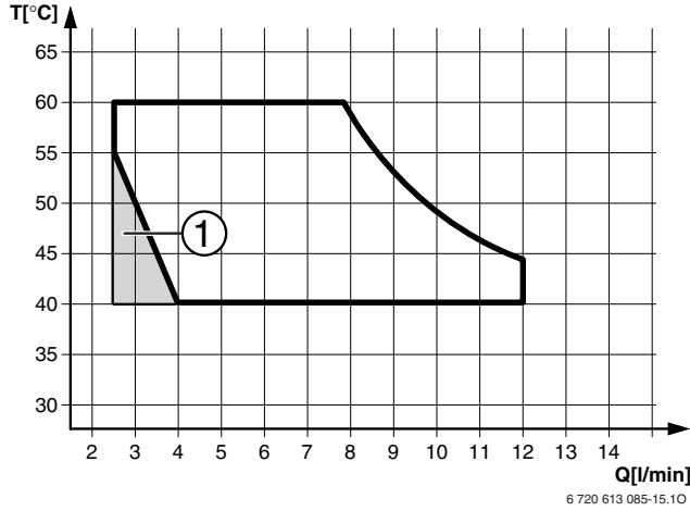
Res. 27 Sıcak Kul. Suyu Performans Diyagramı (Giriş Suyu Sıcaklığı = +15 °C) (B1 RDW 24 21 / ZWC 24-3..)
