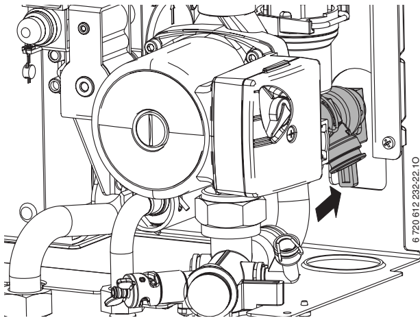
Res. 56 Emniyet Ventili (Isıtma Devresi)
