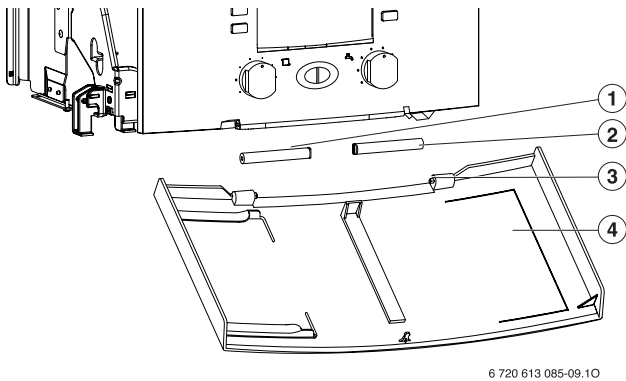
Res. 10 Ön Kapak Montajı
