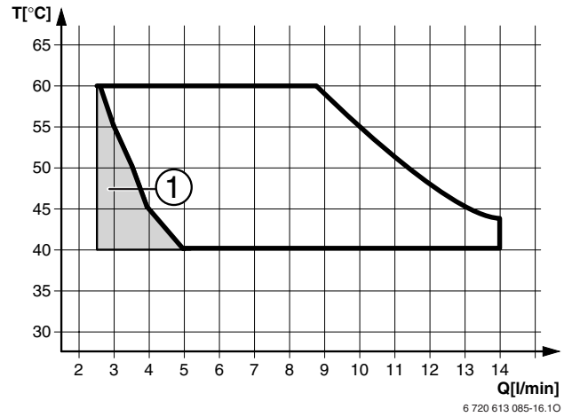
Res. 28 Sıcak Kul. Suyu Performans Diyagramı (Giriş Suyu Sıcaklığı = +15 °C) (B1 RDW 28 21 / ZWC 28-3..)
