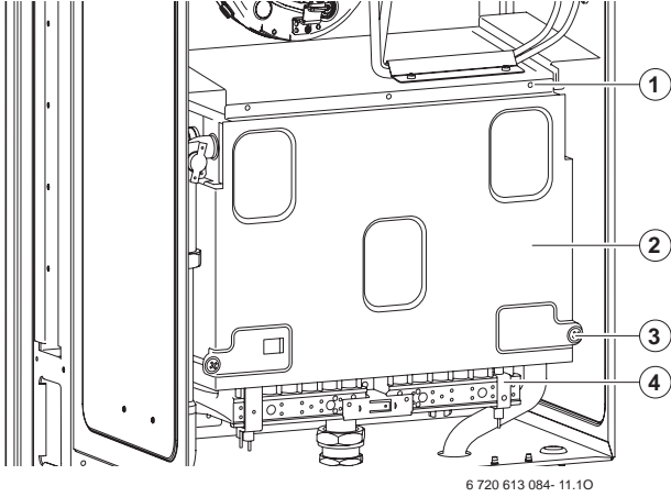
Res. 47 Yanma Odası Kapağının Sökülmesi
