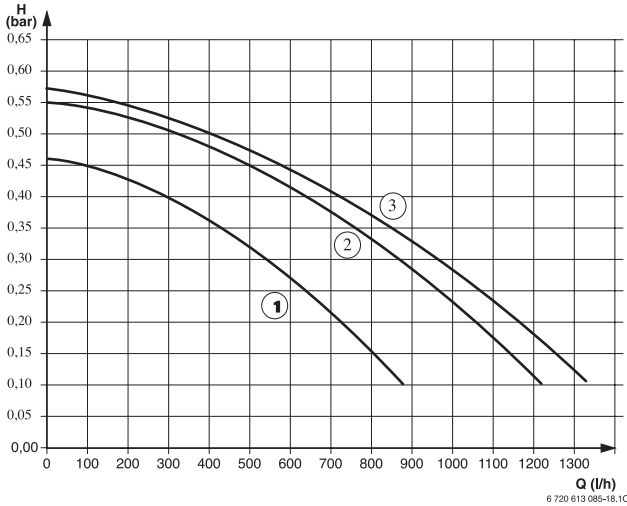
Res. 34 Isıtma Pompası Karakteristik Eğrisi - 28 kW
