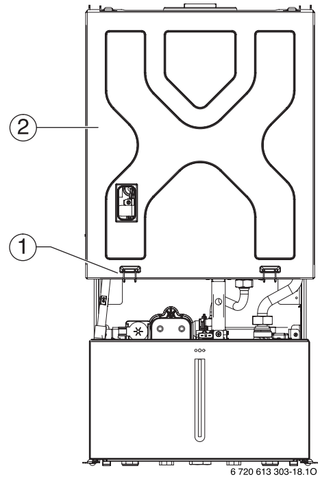
Res. 46 Taze hava kamarası kapağının açılması
