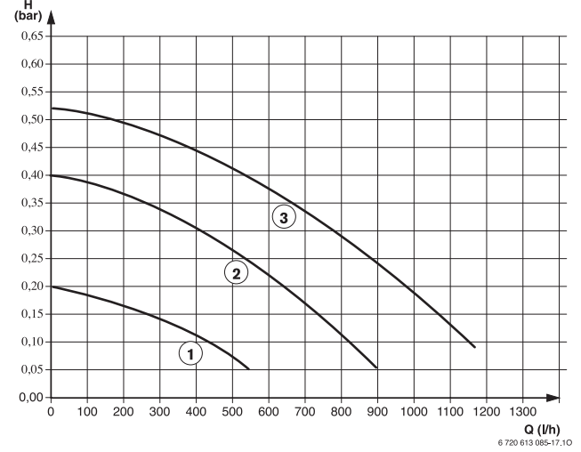
Res. 33 Isıtma Pompası Karakteristik Eğrisi - 24 kW
