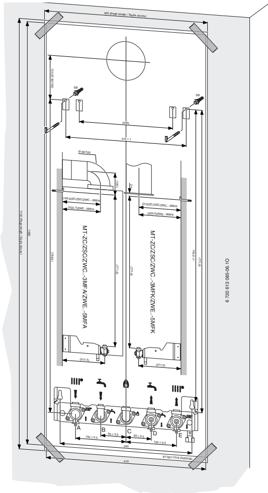
Res. 7 Montaj Şablonu
