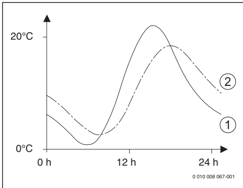
Res. 15 Sönümlenmiş dış hava sıcaklığı için örnek
