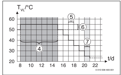
Res. 21 Soğutma aşamasında temel ayarlar ile şap kurutması süreci
