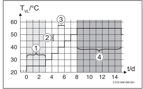
Res. 20 Isıtma aşamasında temel ayarlar ile şap kurutması süreci
