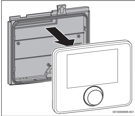
Res. 12 Montaj çerçevesini kumanda panelinin arka tarafına yerleştirin
