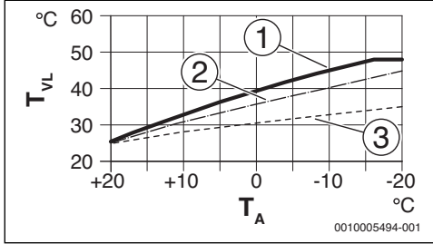
Res. 16 Yerden ısıtma sistemi için ısıtma eğrisinin ayarı Tasarım sıcaklığı T_{AL} ve minimum dış hava sıcaklığı T_{A,min} üzerinden yukarı eğilim
