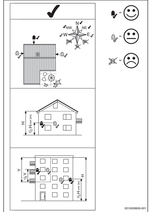
Res. 13 Uygun dış hava sıcaklığı sensörü pozisyonu
