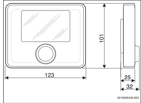
Res. 4 Ölçüler mm olarak belirtilmiştir
