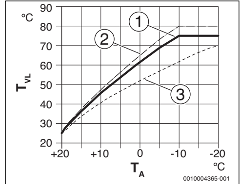
Res. 18 Radyatör için ısıtma eğrisinin ayarı Tasarım sıcaklığı T_{AL} ve minimum dış hava sıcaklığı T_{A,min} üzerinden yukarı eğilim
