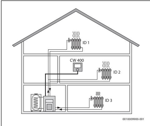
Res. 1 C 400/C 800, birden fazla ısıtma devresi (burada üç) için kumanda cihazı olarak kullanılır
