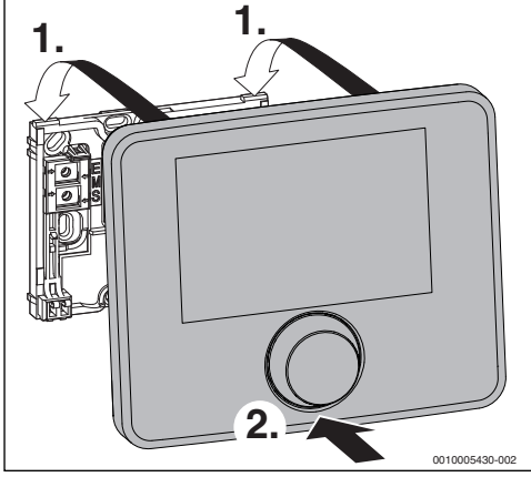
Res. 8 Kumanda panelinin asılması
