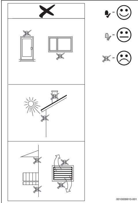
Res. 14 Uygun olmayan dış hava sıcaklığı sensörü pozisyonu
