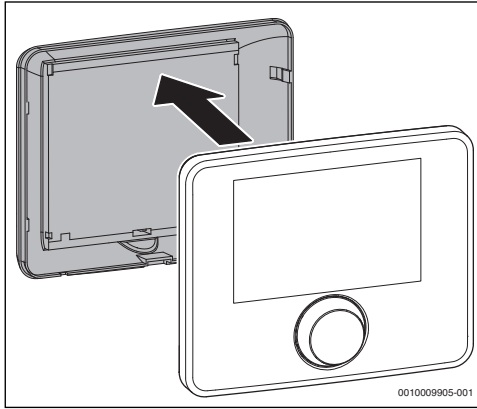
Res. 11 Kumanda panelinin arka tarafındaki kapağı çıkarın
