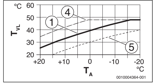
Res. 17 Yerden ısıtma sistemi için ısıtma eğrisi ayarı Oda sıcaklığı ofseti veya istenen oda sıcaklığı üzerinden paralel öteleme
