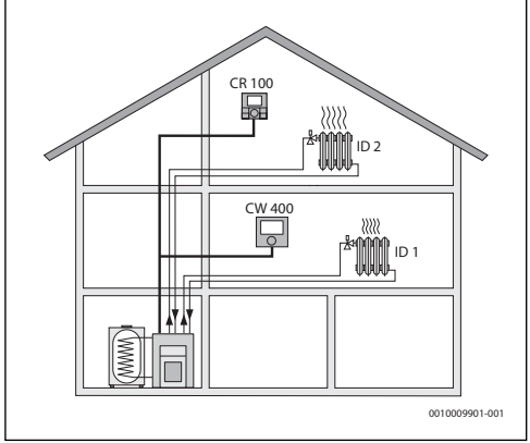
Res. 2 CR 100, ikinci ısıtma devresinde (HK 2) uzaktan kumanda ve C 400/C 800, birinci ısıtma devresinde (HK 1) kumanda cihazı olarak kullanılır
