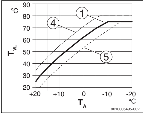
Res. 19 Radyatör için ısıtma eğrisi ayarı Oda sıcaklığı ofseti veya istenen oda sıcaklığı üzerinden paralel öteleme
