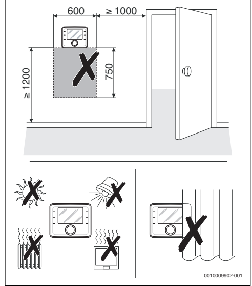
Res. 5 Referans odasındaki montaj yeri
