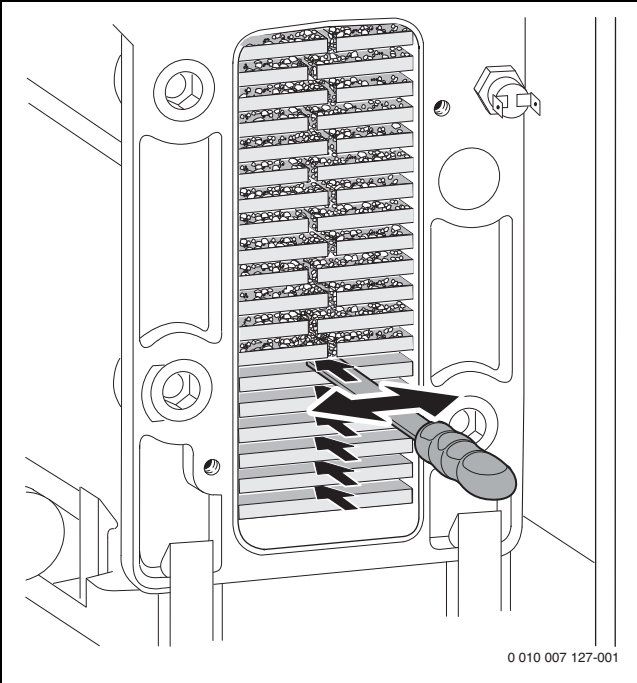
Res. 19 Temizleme bıçağı
