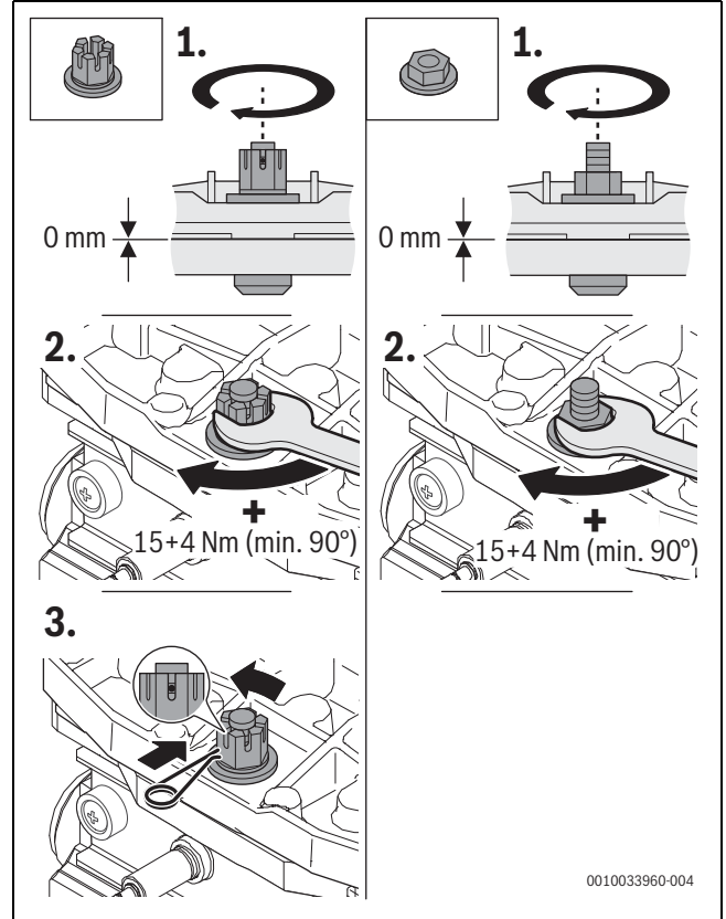
Res. 16 Brülör kapağındaki somunun sıkılması
