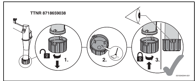
Res. 24 Pislik tutucunun temizlenmesi
