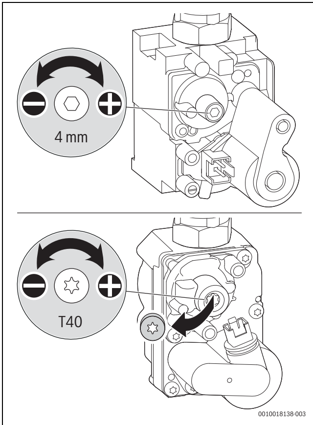
Res. 9 CO 2 veya O 2 miktarının ayarlanması
