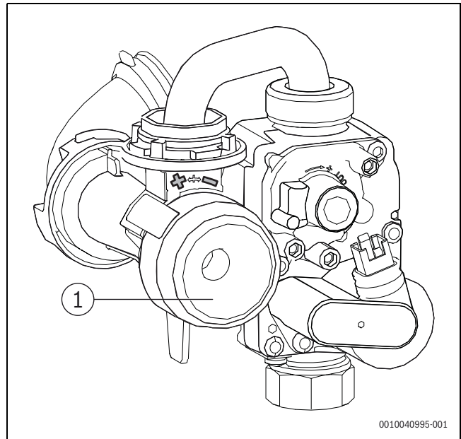
Res. 7 Gaz/hava oranının kontrol ayarlanması
