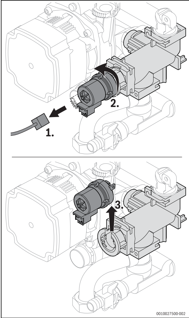
Res. 28 3 yollu vana motorunun sökülmesi (civatasız model)
