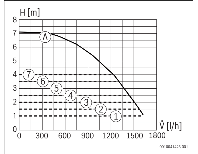
Res. 32 Pompa karakteristik alanları ve pompa karakteristik eğrileri
