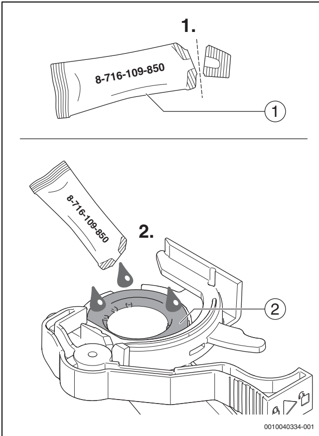
Res. 26 Contanın greslenmesi
