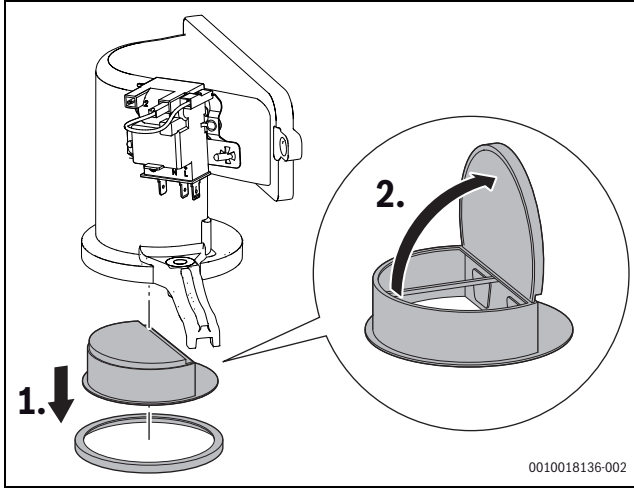
Res. 18 Karıştırma ünitesindeki çekvalf
