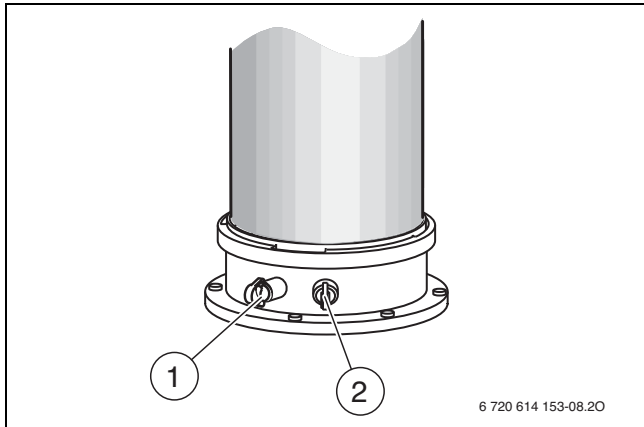
Res. 11 Atık gaz ölçüm bağlantısı ve yanma havası ölçüm bağlantısı
