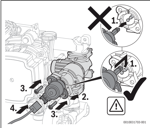
Res. 31 Motorun 3 yollu vanaya monte edilmesi (civatalı model)
