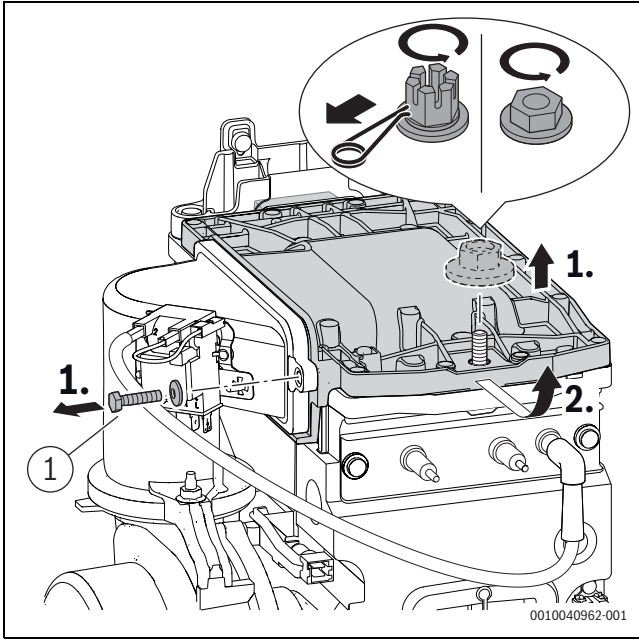
Res. 14 Brülör kapağının sökülmesi
