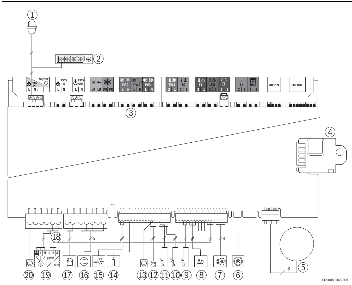
Res. 33 Elektrik bağlantısı
