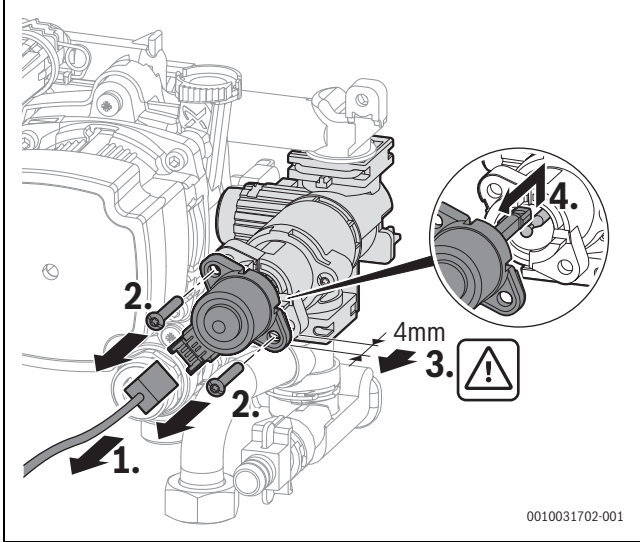
Res. 30 3 yollu vana motorunun sökülmesi (civatalı model)
