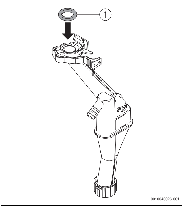
Res. 25 Yeni contanın yoğuşma suyu sifonuna takılması
