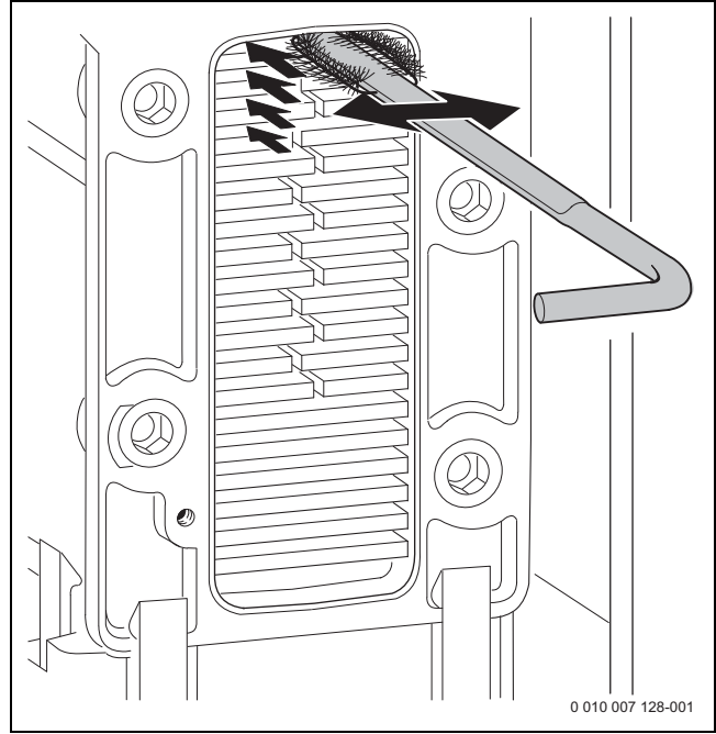
Res. 20 Isı bloğunun fırça ile temizlenmesi
