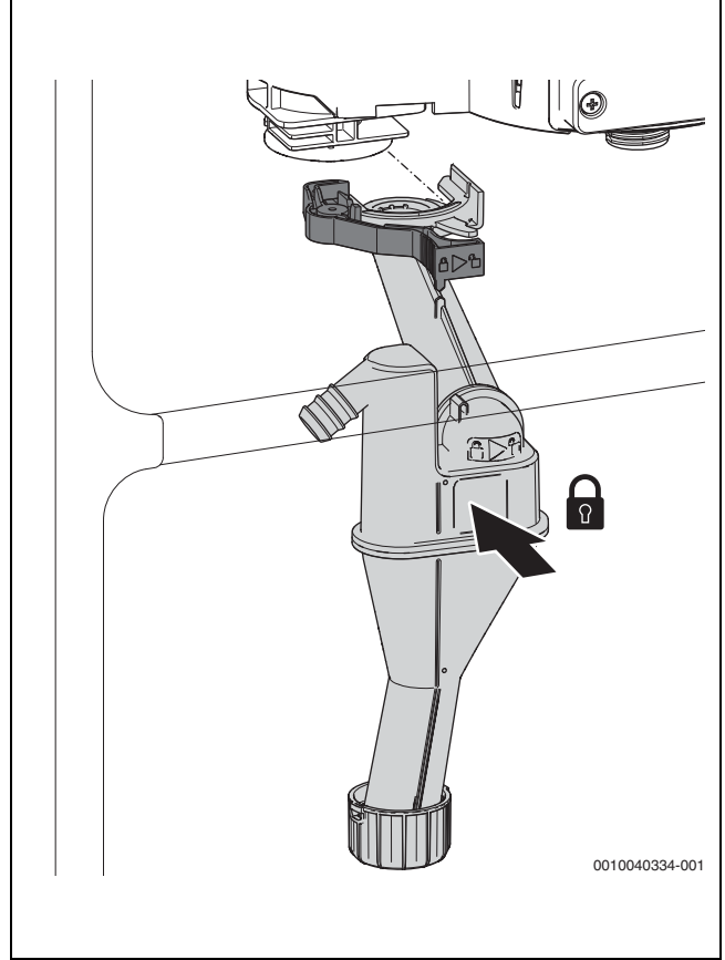
Res. 27 Yoğuşma suyu sifonunun takılması
