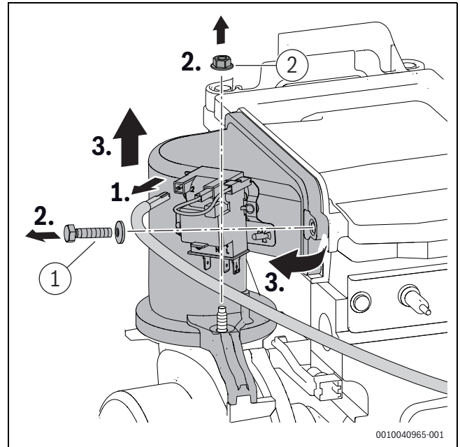
Res. 17 Karıştırma ünitesinin sökülmesi
