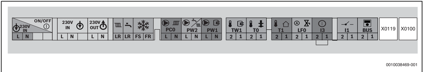
Res. 5 Harici aksesuar için terminal bloğu
