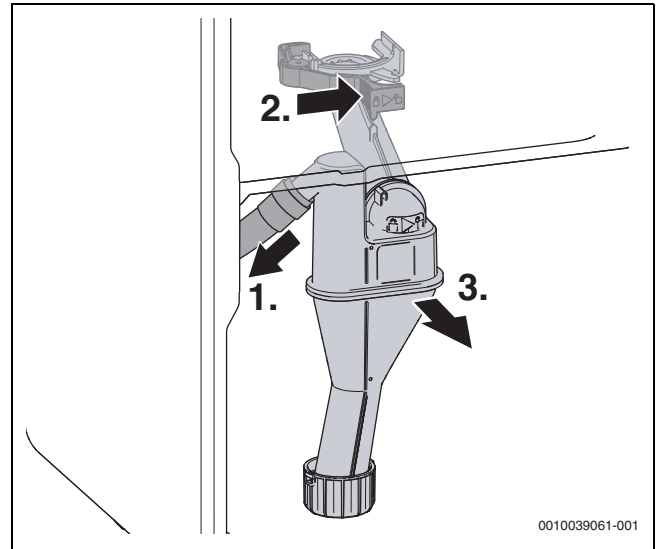
Res. 23 Yoğuşma suyu sifonunun sökülmesi
