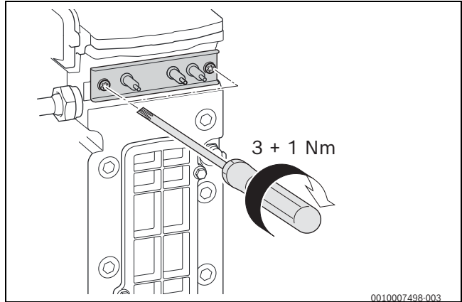
Res. 12 Elektrotlar setinin monte edilmesi
