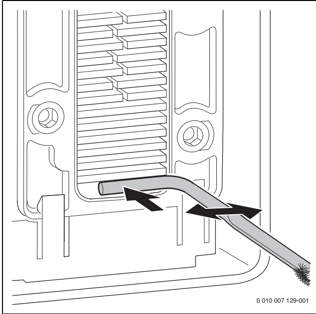
Res. 22 Yoğuşma suyu kabının temizlenmesi
