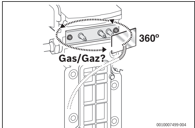
Res. 13 Sızdırmazlık kontrolü
