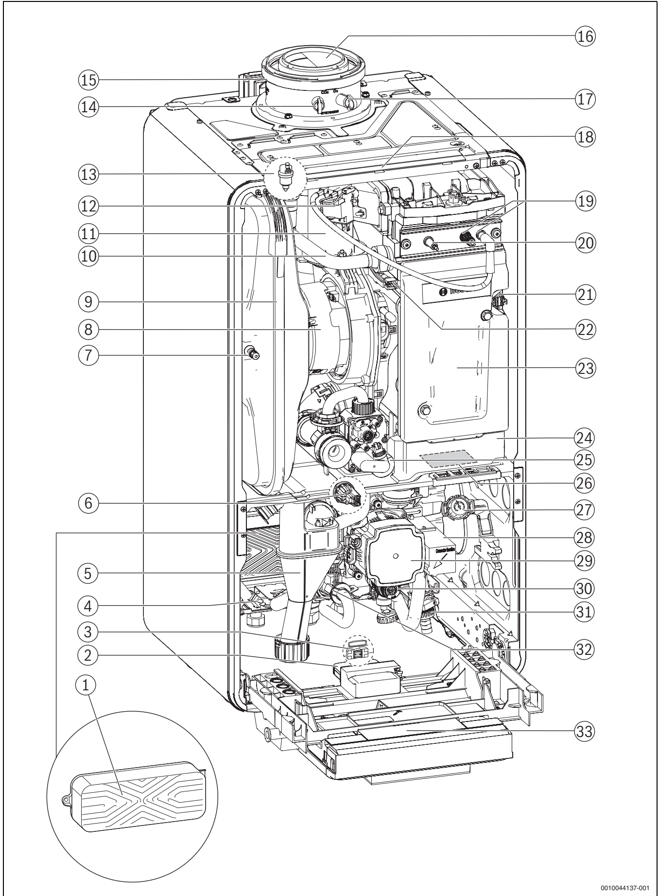
Res. 1 Ürüne genel bakış - Kombi cihazı
