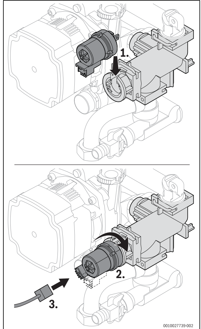
Res. 29 Motorun 3 yollu vanaya monte edilmesi (civatasız model)
