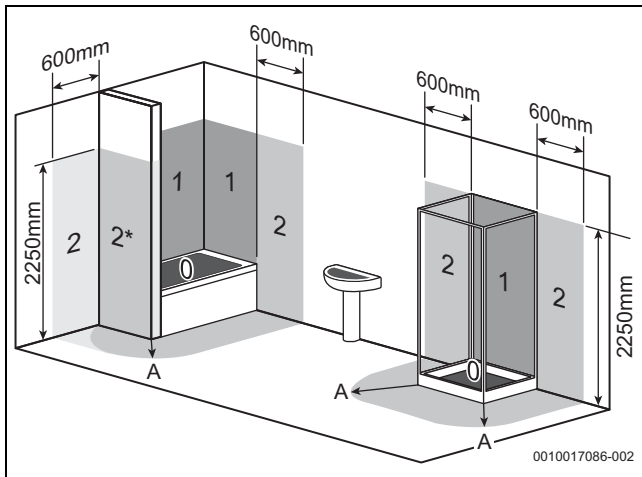
Res. 22 Koruma alanları (örnek gösterim)
