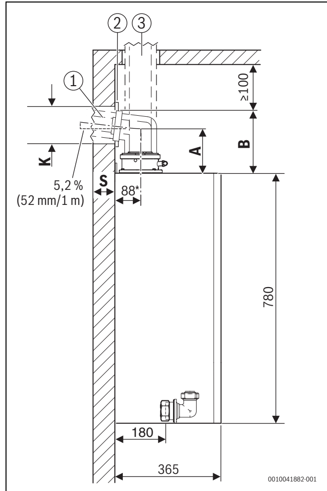
Res. 4 Yandan görünüm (mm)
