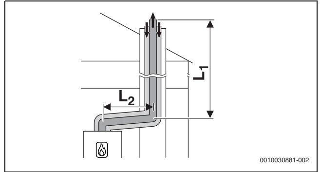
Res. 11 Havalandırma boşluğunda C 33x uyarınca konsantrik hava-atık gaz taşıma sistemi
