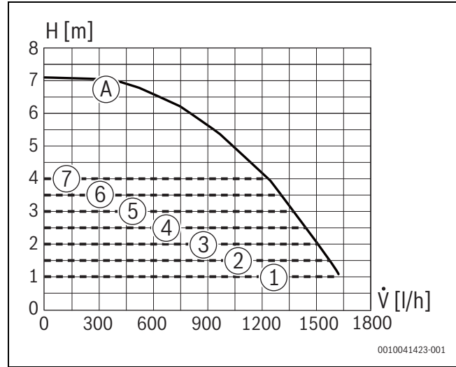
Res. 36 Pompa karakteristik alanları ve pompa karakteristik eğrileri
