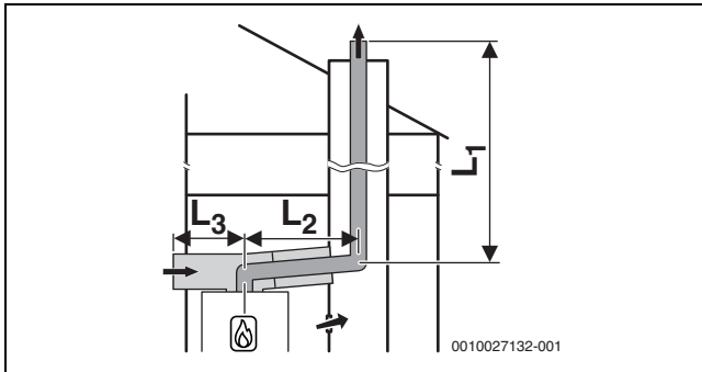
Res. 13 Şaftta ve ayrı hava beslemeli hava-atık gaz taşıma sisteminde C 53x uyarınca sabit atık gaz tahliyesi ve kazan dairesinde konsantrik atık gaz hattı
