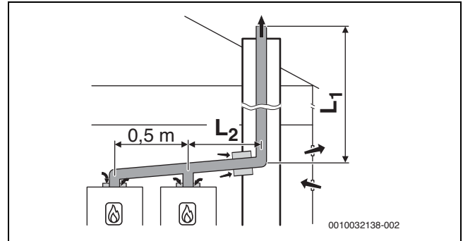
Res. 20 2 cihaz içeren kaskad:
