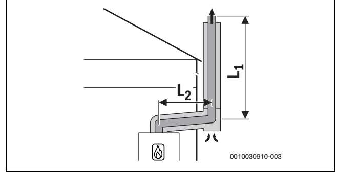
Res. 14 Dış duvar üzerinde C 53x uyarınca konsantrik hava-atık gaz taşıma sistemi
