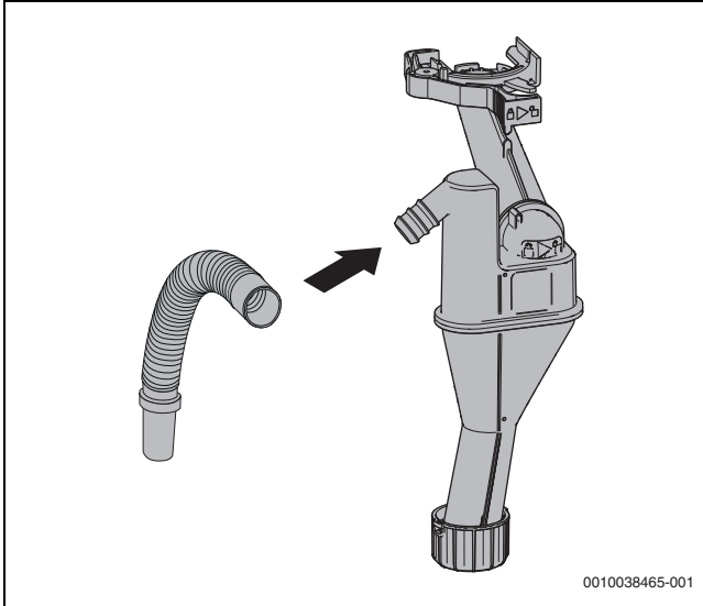
Res. 28 Yoğuşma suyu hortumunun bağlantı parçasına takılması
