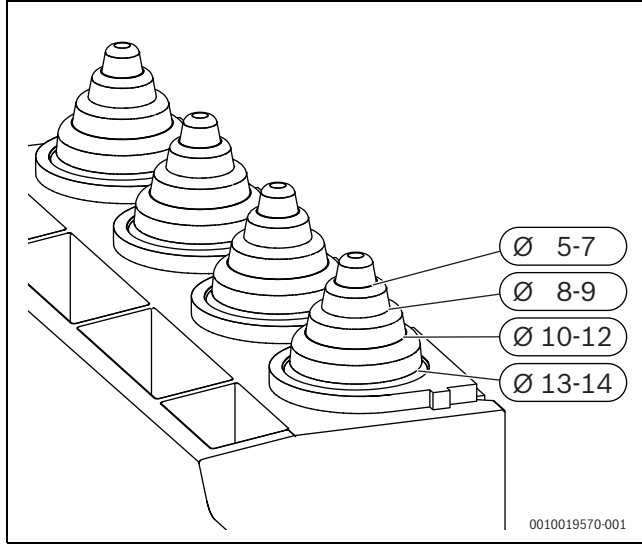
Res. 33 Sabitleme bandının kablo çapına uygun ayarlanması
