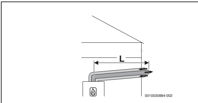
Res. 10 C 13x uyarınca dış duvardan geçen yatay konsantrik hava-atık gaz taşıma sistemi
