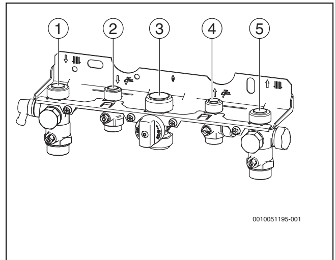
Res. 31 Gaz ve su tarafındaki bağlantılar
