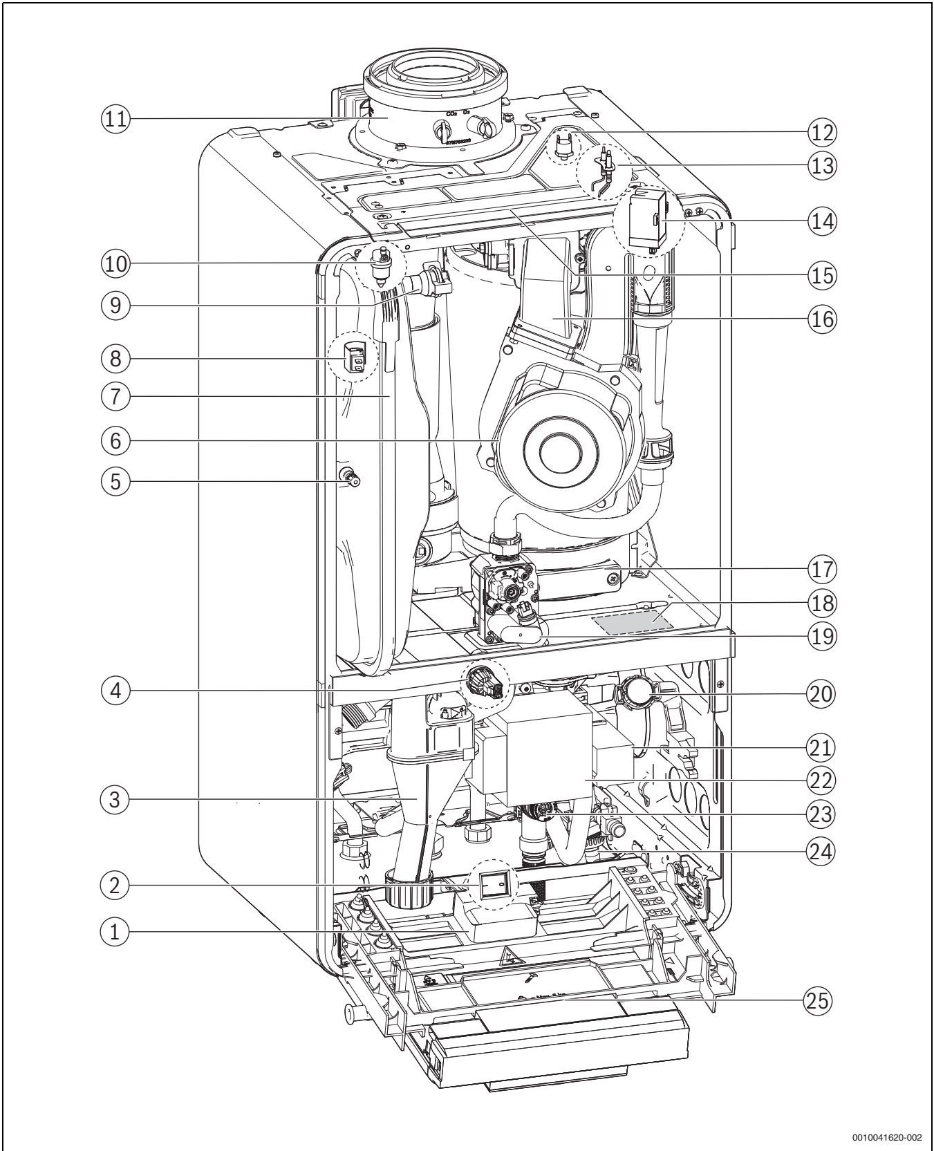
Res. 7 Ürüne genel bakış - Depolu cihaz
