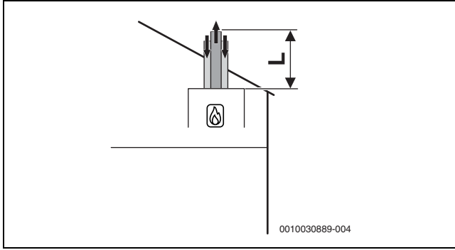
Res. 12 C 33x uyarınca dikey konsantrik hava-atık gaz taşıma sistemi
