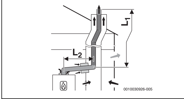
Res. 18 Cihazda oda havasına bağlı hava beslemeli ve kurulum yerinde tek cidarlı atık gaz hattı, havalandırma boşluğunda B 53p uyarınca esnek atık gaz tahliyesi; havalandırma boşluğunda arka havalandırma açıklığı
