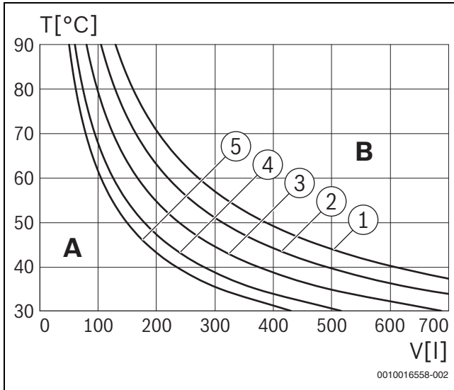
Res. 25 Genleşme tankının karakteristik eğrileri
