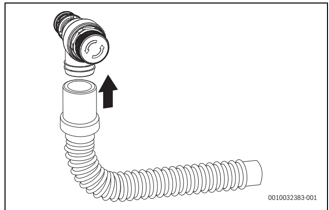
Res. 27 Hortumun emniyet ventiline (ısıtma tesisatı) monte edilmesi
