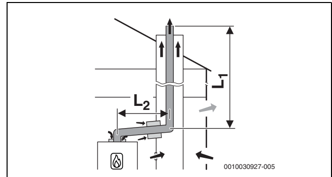
Res. 17 Cihazda oda havasına bağlı hava beslemeli ve kurulum yerinde tek cidarlı atık gaz hattı, havalandırma boşluğunda B 53p uyarınca sabit atık gaz tahliyesi; havalandırma boşluğunda arka havalandırma açıklığı
