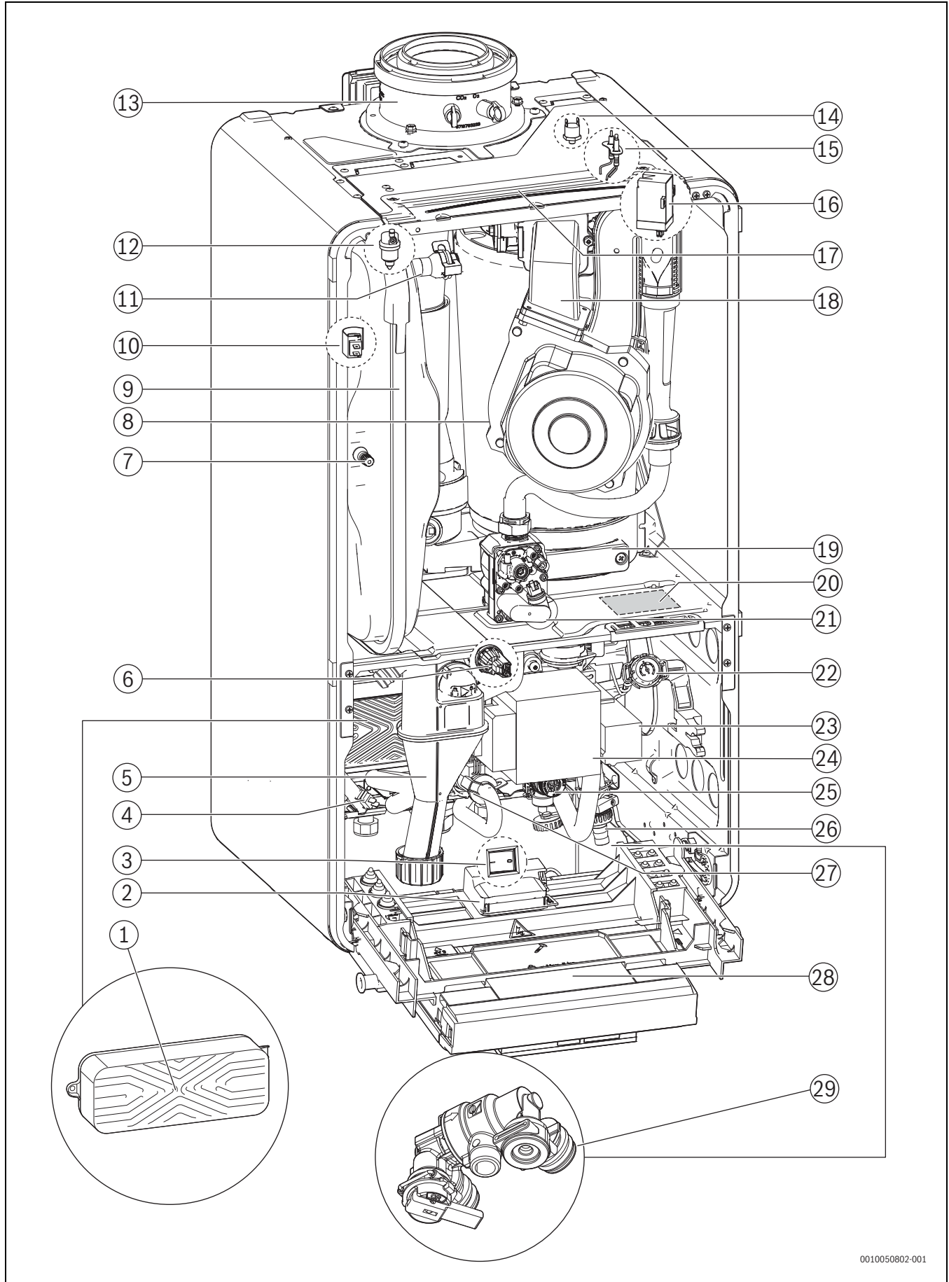
Res. 6 Ürüne genel bakış - Kombi cihazı
