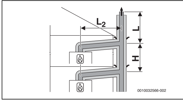
Res. 19 Dış duvarda ve kazan dairesinde konsantrik hava-atık gaz taşıma sistemli C_{(13)3x} uyarınca çoklu bağlantı
