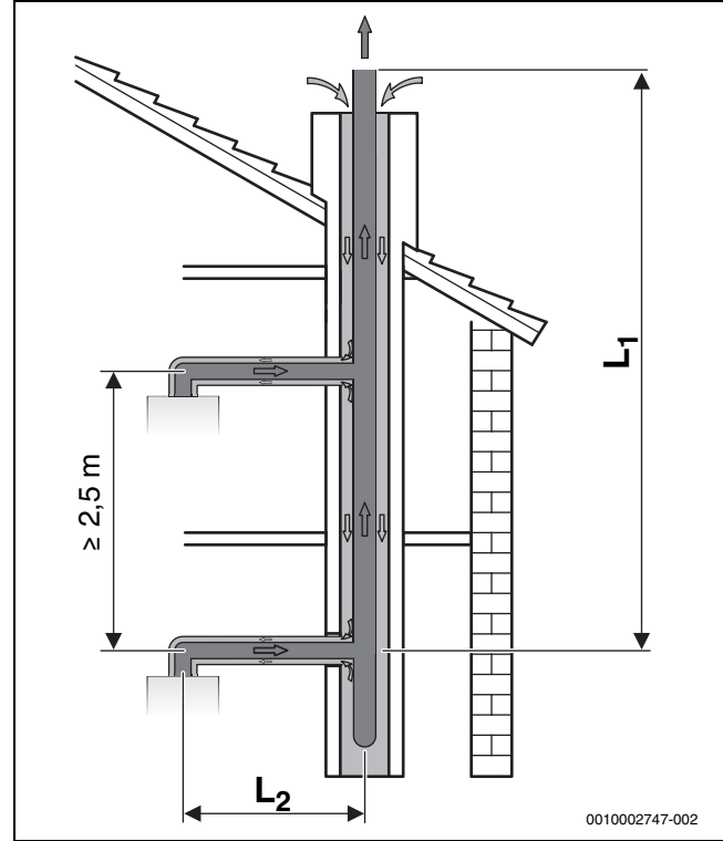
Res. 18 C 43(x) 'e uygun olarak konsantrik boru ile çoklu kullanım
