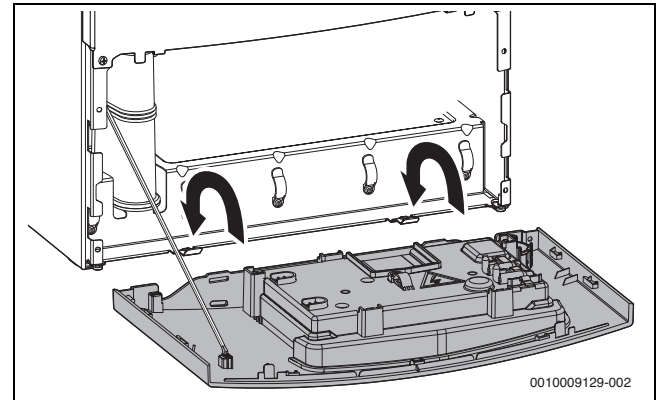
Res. 24 Kumanda cihazını servis pozisyonuna getirme
