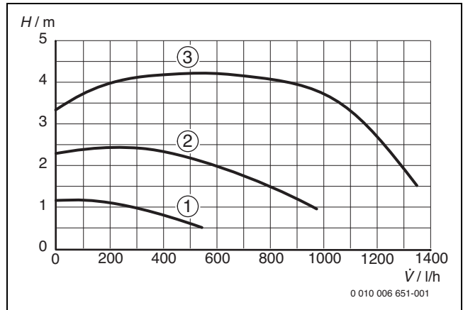
Res. 39 Sirkülasyon pompasının karakteristik eğrisi (modülasyonlu hız)
