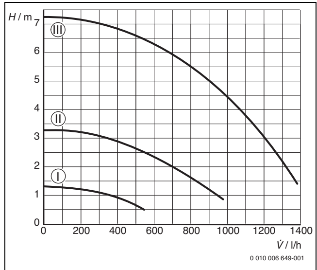
Res. 38 Sirkülasyon pompası karakteristik eğrisi (sabit hız)
