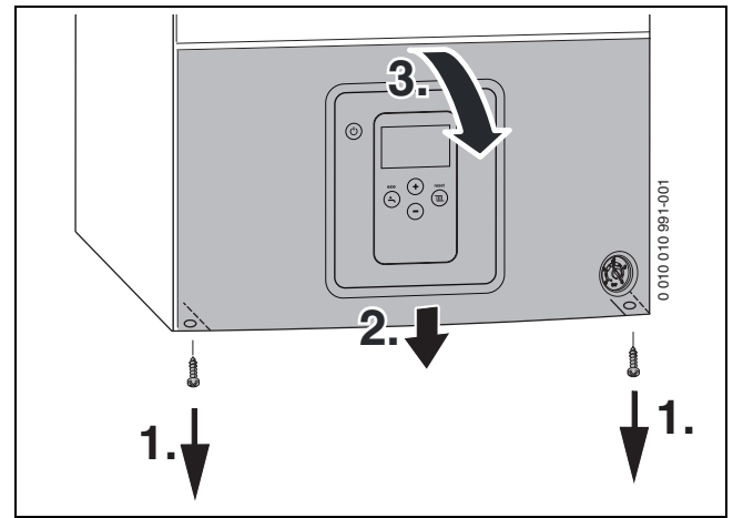
Res. 23 Kumanda cihazının aşağı doğru açılması
