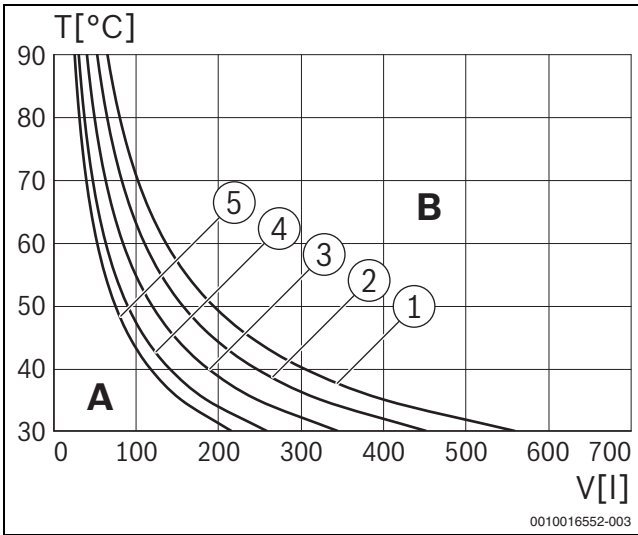
Res. 22 Genleşme tankının karakteristik eğrileri
