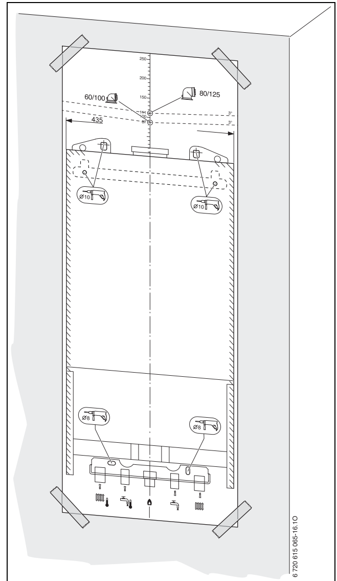
Bild 10 Montaj Şablonu
