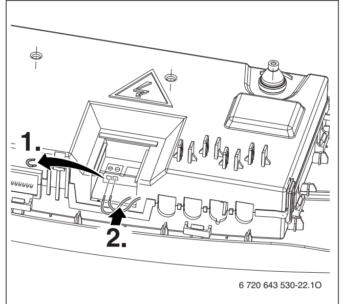
Res. 14 Oda Termostatı Bağlantısı (230 VAC veya OT, TH soketindeki köprü çıkartılmalıdır)
