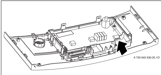
Res. 16 230V Şebeke Kablosu Bağlantısı
