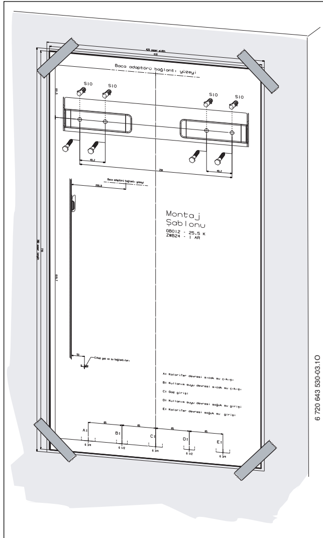
Res. 6 Montaj Şablonu
