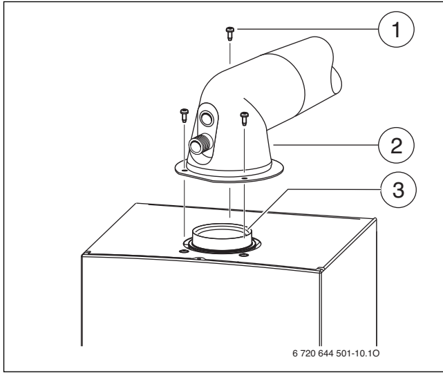
Res. 10 Atık Gaz Tahliye Aks. Montajı
