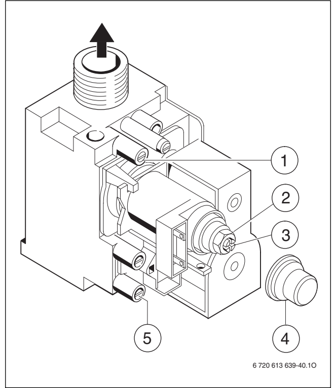
Res. 30 Gaz Armatürü
