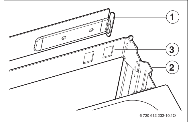
Res. 7 Cihazın askı sacına takılması
