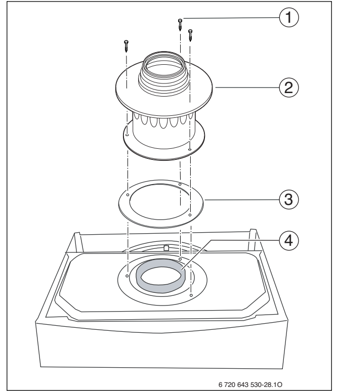
Res. 11 B 22 Tipi Atık Gaz Tahliyesi
