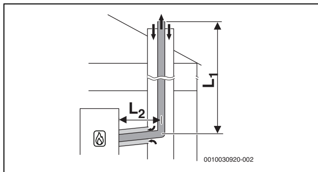
Res. 10 Havalandırma boşluğunda C 93x uyarınca sabit atık gaz tahliyesi ve kurulum yerinde konsantrik hava-atık gaz taşıma sistemi
