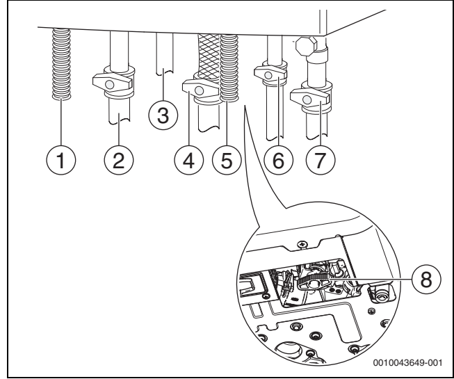
Res. 19 Gaz ve su tarafındaki bağlantılar (aksesuar)
