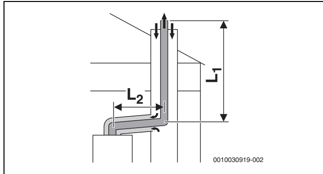
Res. 9 Havalandırma boşluğunda C 93x uyarınca sabit atık gaz tahliyesi ve kurulum yerinde konsantrik hava-atık gaz taşıma sistemi
