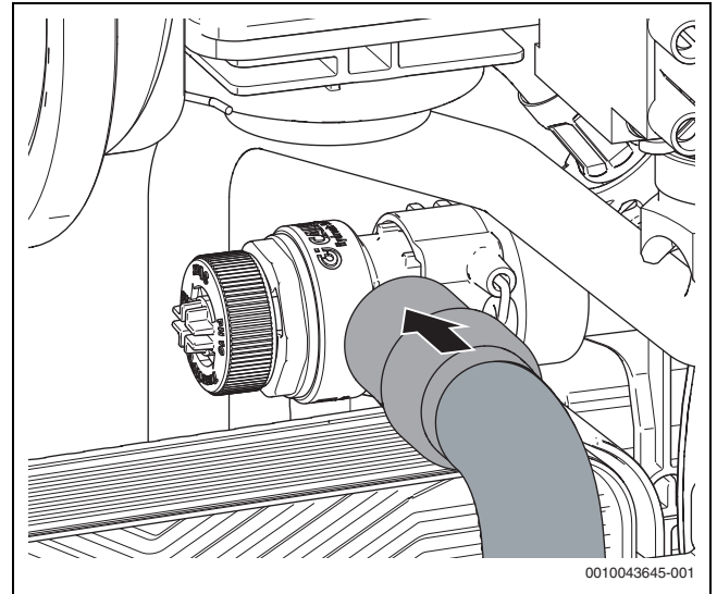
Res. 17 Hortumun emniyet ventiline monte edilmesi
