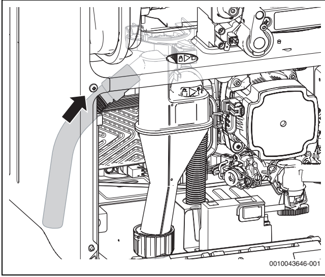
Res. 18 Hortumun yoğuşma suyu sifonuna monte edilmesi
