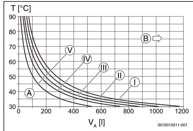
Res. 15 Genleşme tankının karakteristik eğrileri
