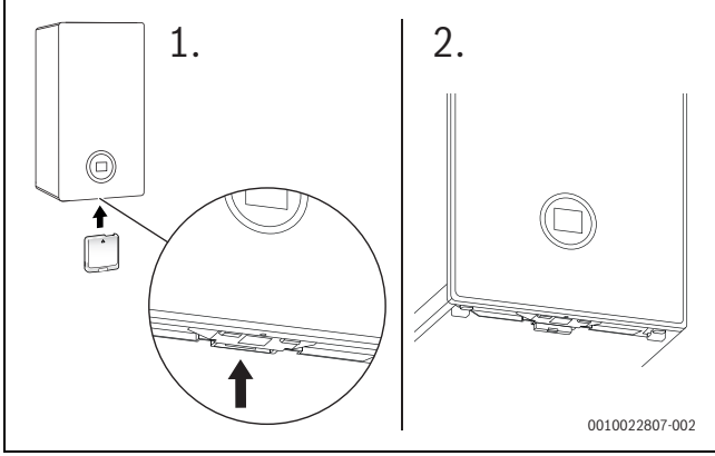
Res. 3 Key soket yuvasının konumu
